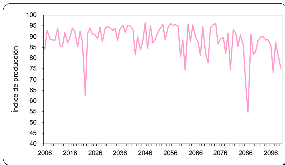
Gráfico 19 EL SALVADOR: PROYECCIONES DEL ÍNDICE PRODUCCIÓN AGRÍCOLA A PARTIR DEL ESCENARIO B2
